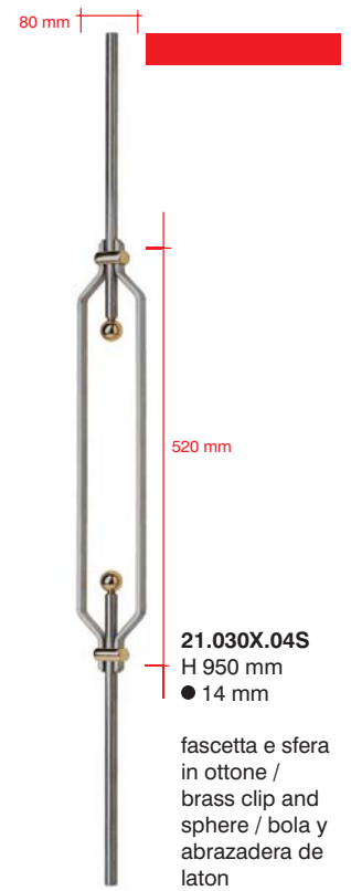
fascetta e sfera in ottone / brass clip and sphere / bola y abrazadera de laton
